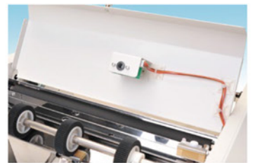
双张检测电眼监测纸张输送过程，防止双张输纸，保证成品质量
